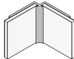
Rohové řešení s vnitřním profilem
