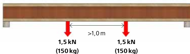
Příklad bodového zatížení
